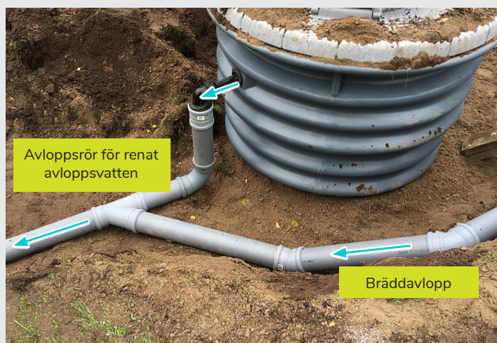
Bild 21: Brøddavlopp och avlopp för renat avloppsvatten
