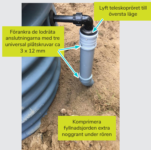
Bild 20: Anslutning av avloppsrör för utgående renat vatten
