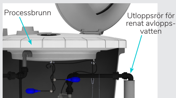
Bild 19: Anslutningskoppling för renat avloppsvatten
