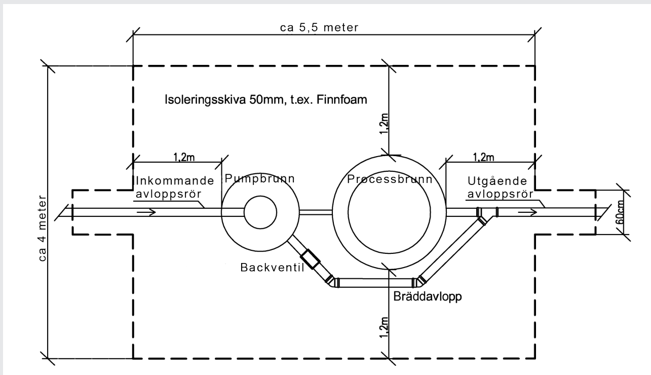
Bild 24: Område för isolering, sett uppifrån
