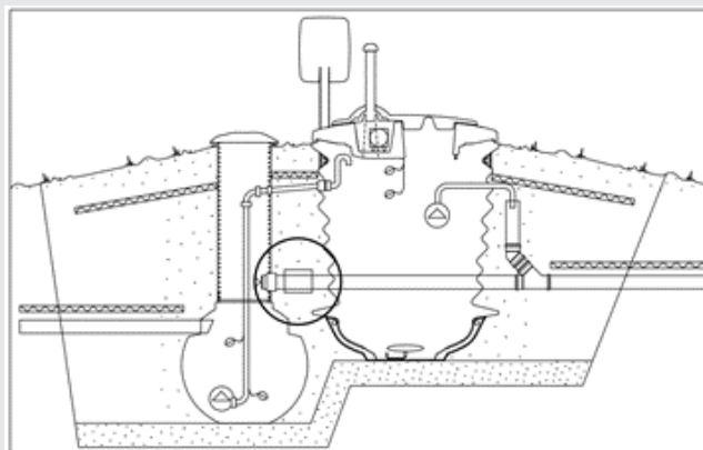
Bild 18: Bräddavlopp och backventil
