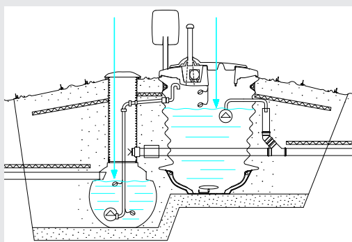
Bild 11: Vattenfyllning
