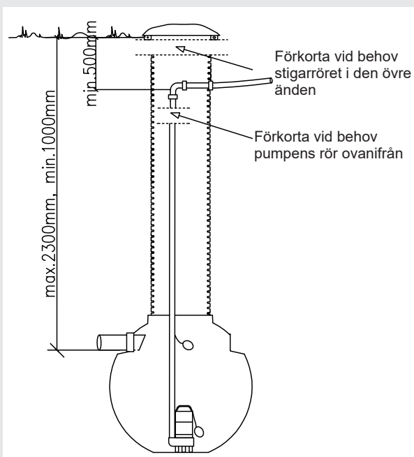
Bild 17: Höjdjustering av pumpbrunnens stigarrör
