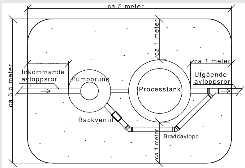
Bild 1: Schaktets mått
