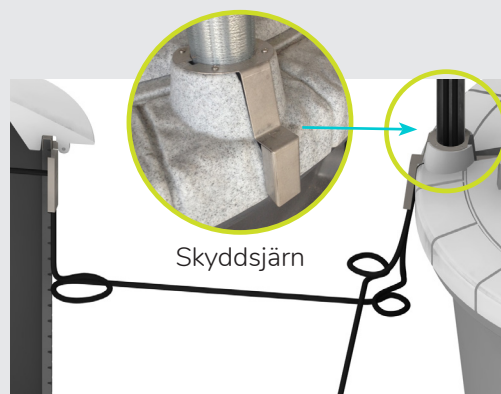
Bild 22: Jordkabel och skyddsjärn
