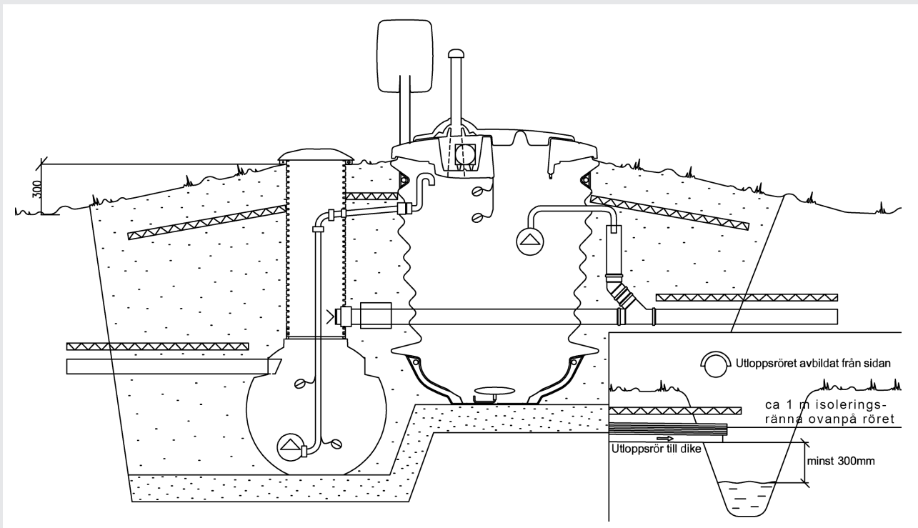
Bild 23: Byggande av en jordkulle
