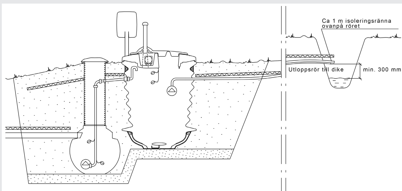
Bild 28: Trycktömning i stigande terräng
