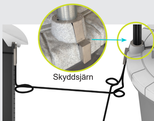
Bild 10: Jordkabel och skyddsjärn
