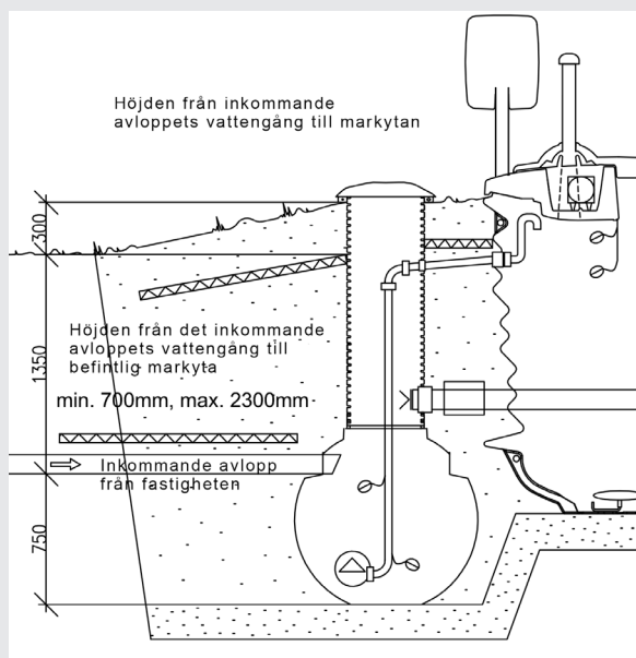
Bild 2: Schaktets djup
