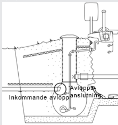
Bild 8: Anslut inkommande avlopp till pumpbrunnen
