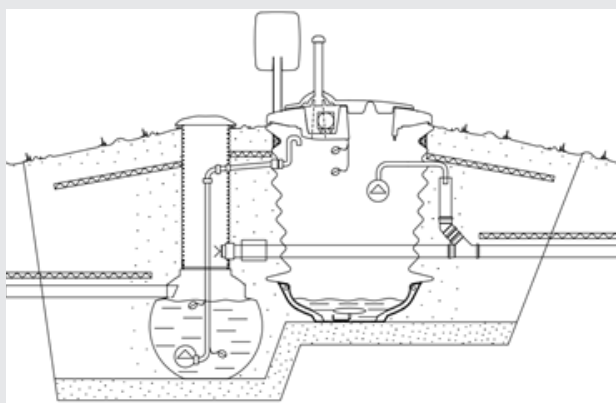
Bild 9: Förfyllt schakt
